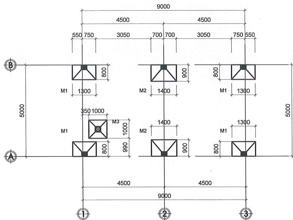
MẶT BẰNG MÓNG TL: 1/100
