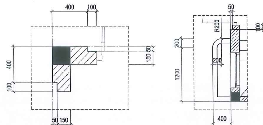
CHI TIẾT 1 TL:1/25
