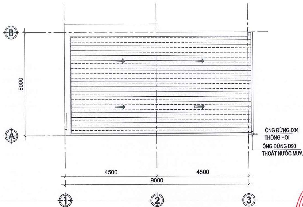
MẶT BẰNG THOÁT NƯỚC MÁI TL: 1/100
