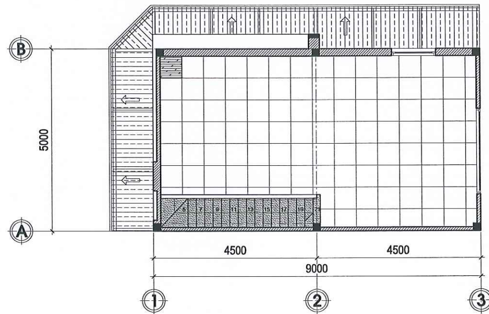
MẶT BẰNG LÁT GẠCH TẦNG 2 TL:1/100
