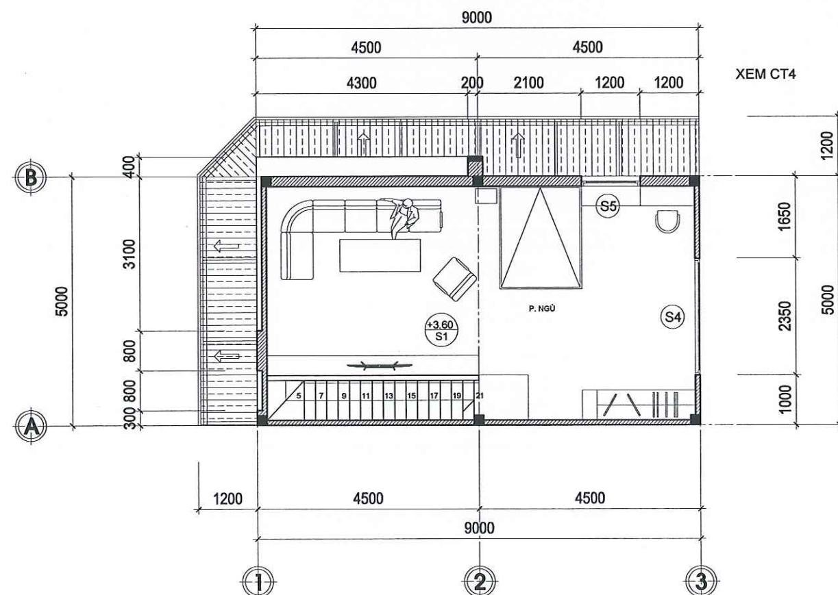
MẶT BẰNG TẦNG 2 TL:1/100
