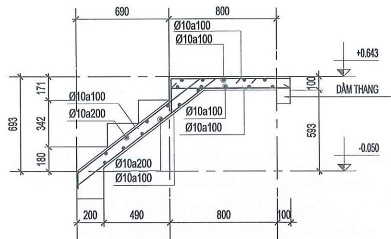
VẾ 1 TL:1/25
