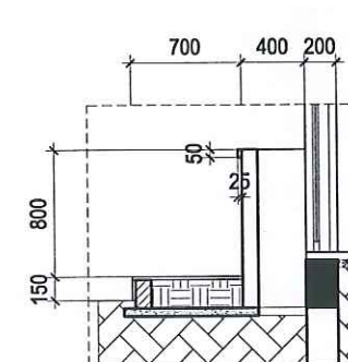
CHI TIẾT 18 TL:1/25
