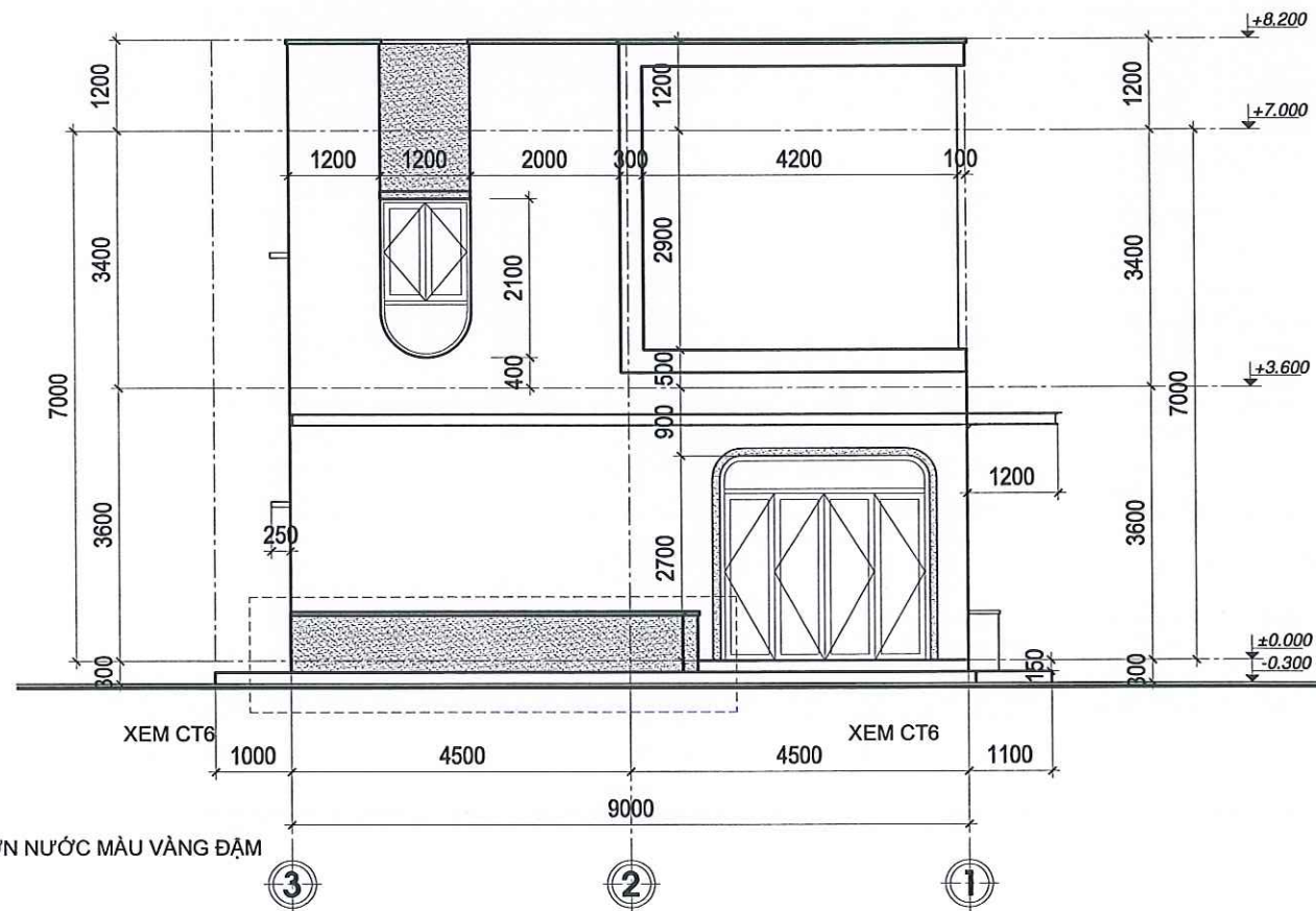
MẶT BẰNG ĐỨNG TRỤC 3-1 TL:1/100
