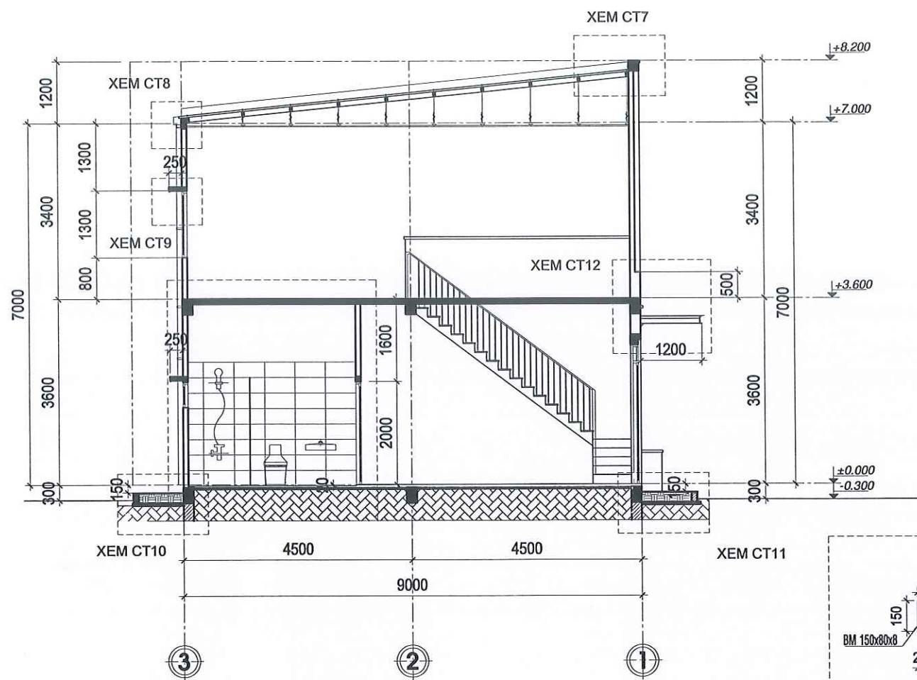
MẶT CẮT 1-1 TL:1/100
