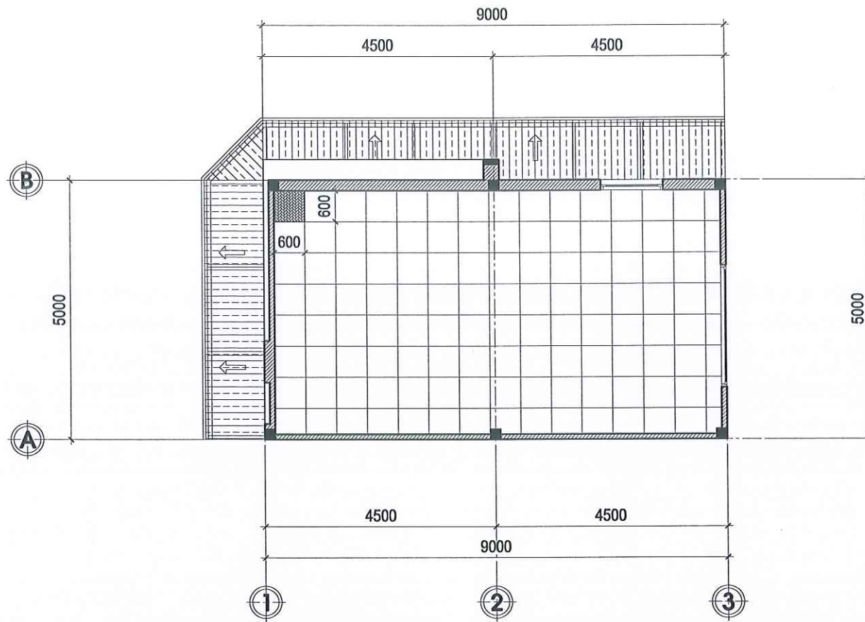
MẶT BẰNG TRẦN THẠCH CAO KHUNG NỔI TẦNG 2 TL:1/100
