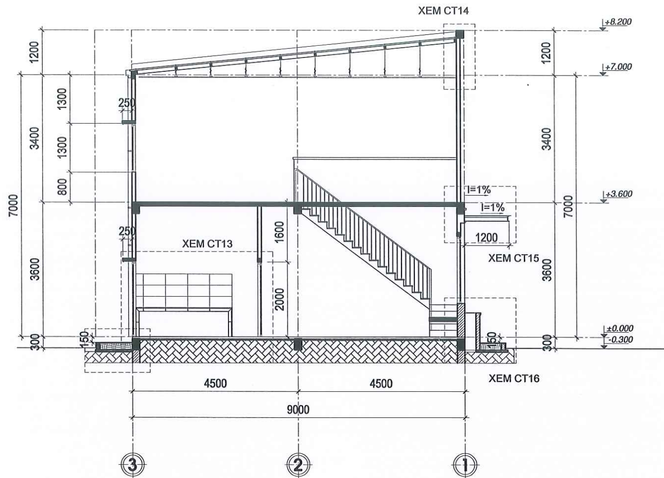
MẶT CẮT 2-2 TL:1/100
