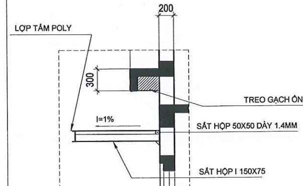
CHI TIẾT 16 TL:1/50
