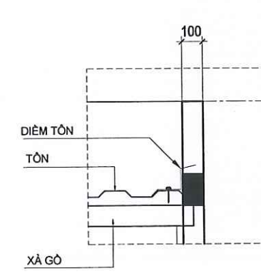
CHI TIẾT 18 TL:1/25
