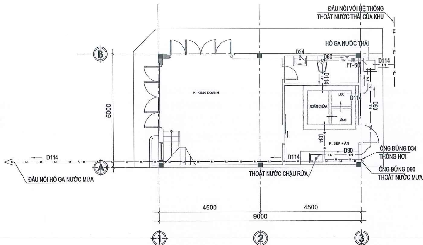
MẶT BẰNG THOÁT NƯỚC TẦNG 1 TL: 1/100
