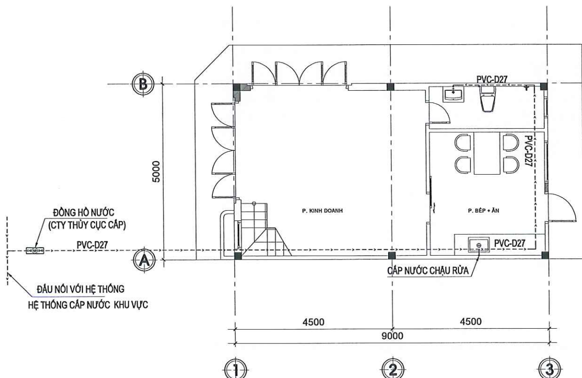
MẶT BẰNG CẤP NƯỚC TẦNG 1 TL: 1/100
