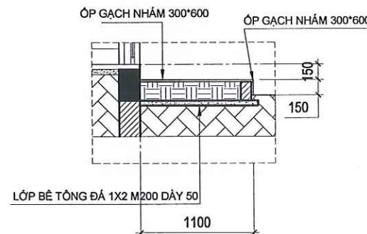
CHI TIẾT 11 TL:1/50
