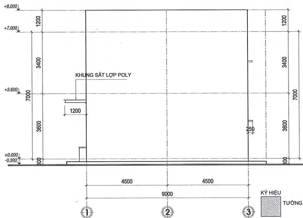
MẶT BẰNG ĐỨNG TRỤC 1-3 TL:1/100
