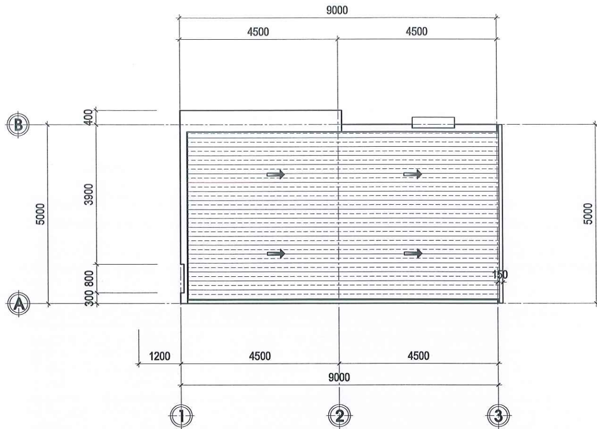
MẶT BẰNG MÁI TL:1/100
