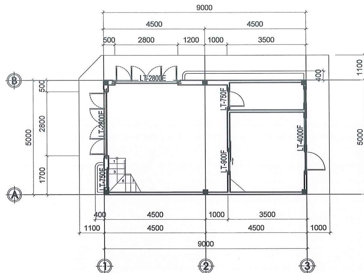
MẶT BẰNG LANH TÔ TẦNG 1
