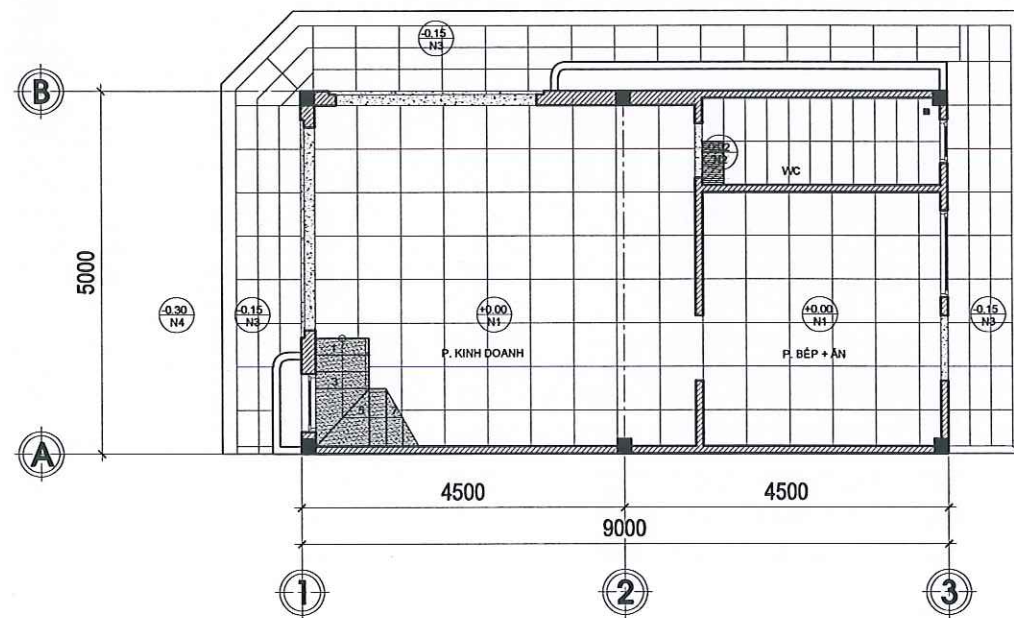
MẶT BẰNG LÁT GẠCH TẦNG 1 TL:1/100
