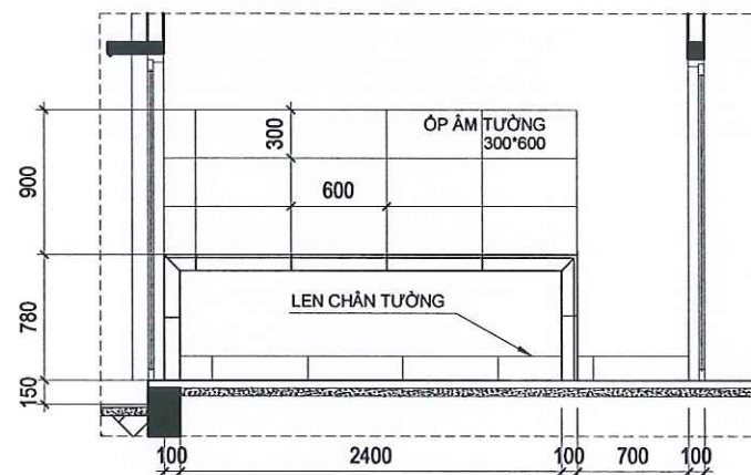
CHI TIẾT 13 TL:1/50
