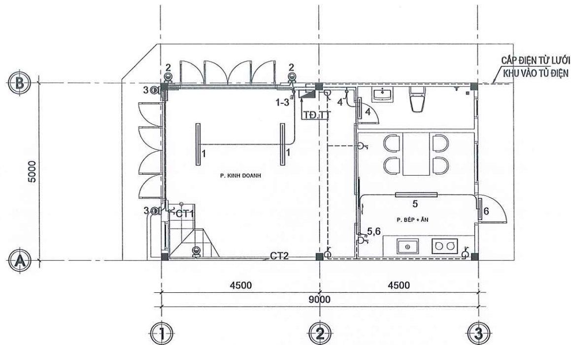
MẶT BẰNG ĐIỆN TẦNG 1 TL: 1/100
