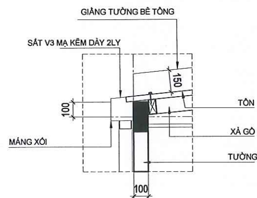
CHI TIẾT 8 TL:1/25
