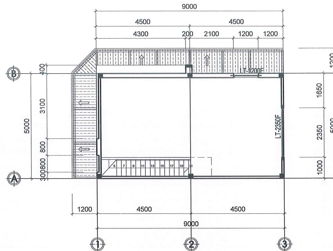
MẶT BẰNG LANH TÔ TẦNG 2
