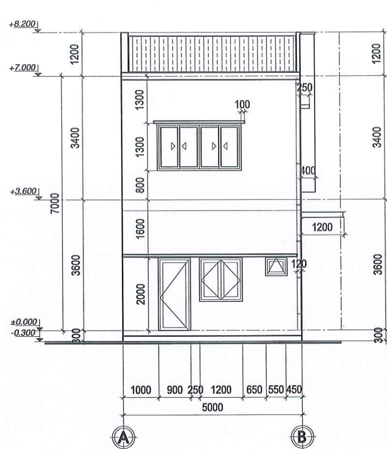
MẶT BẰNG ĐỨNG TRỤC A-B TL:1/100
