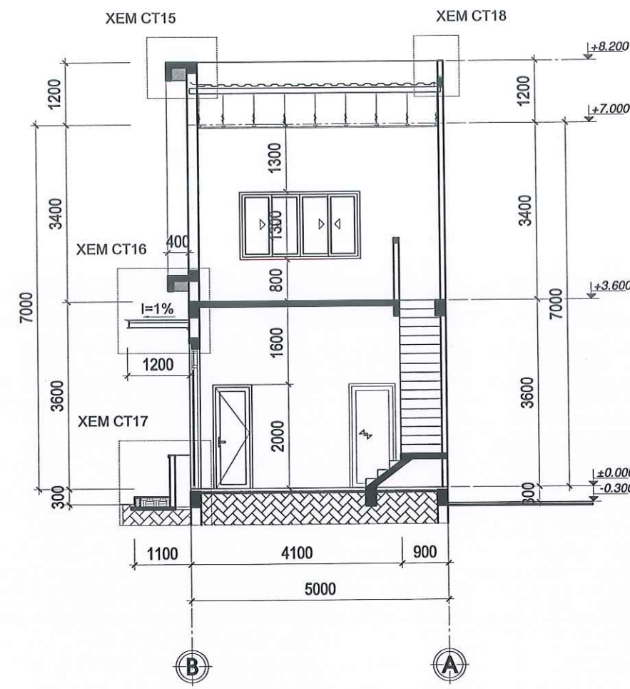
MẶT CẮT 3-3 TL:1/100
