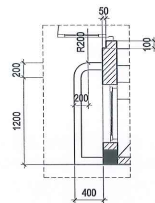
CHI TIẾT 2 TL:1/50
