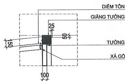
CHI TIẾT 7 TL:1/50
