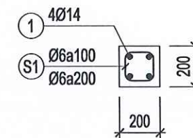
CHI TIẾT CỘT C-1
