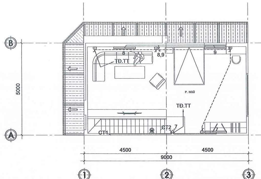
MẶT BẰNG ĐIỆN TẦNG 2 TL: 1/100
