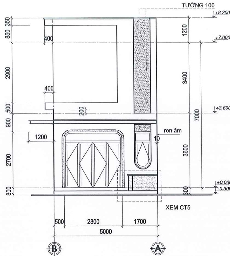
MẶT BẰNG ĐỨNG TRỤC B-A TL:1/100
