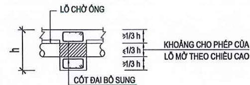
MẶT CẮT X - X
