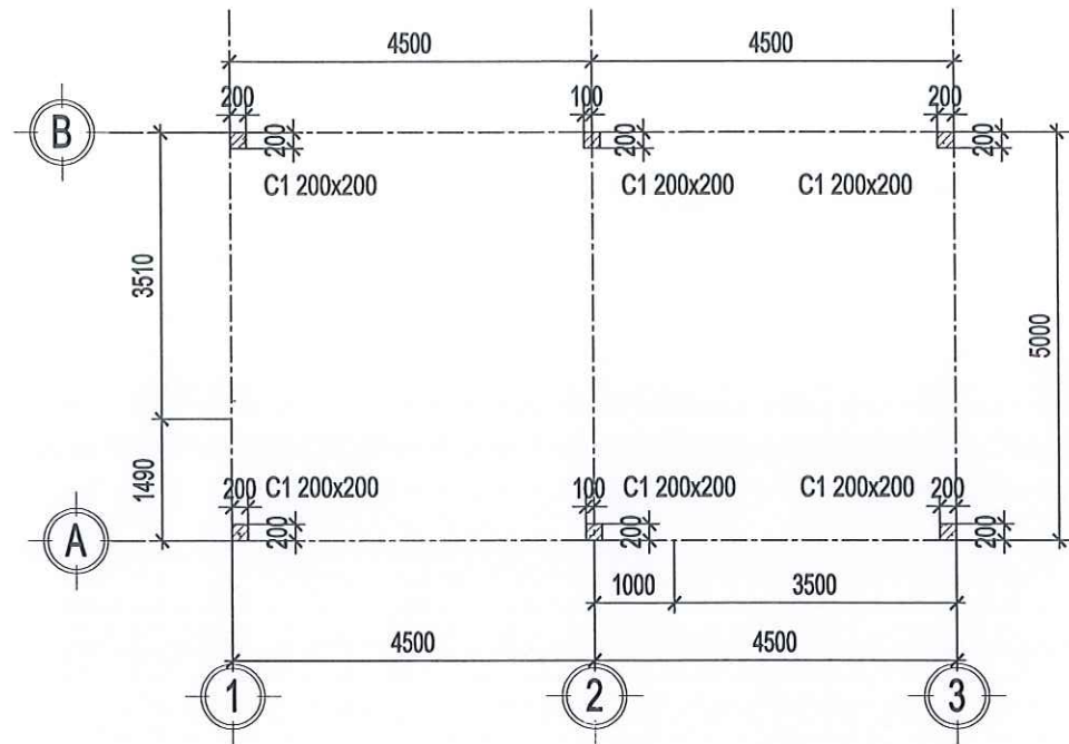
MẶT BẰNG CỘT TẦNG 1
