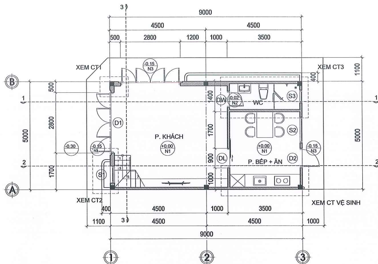
MẶT BẰNG TẦNG 1 TL:1/100
