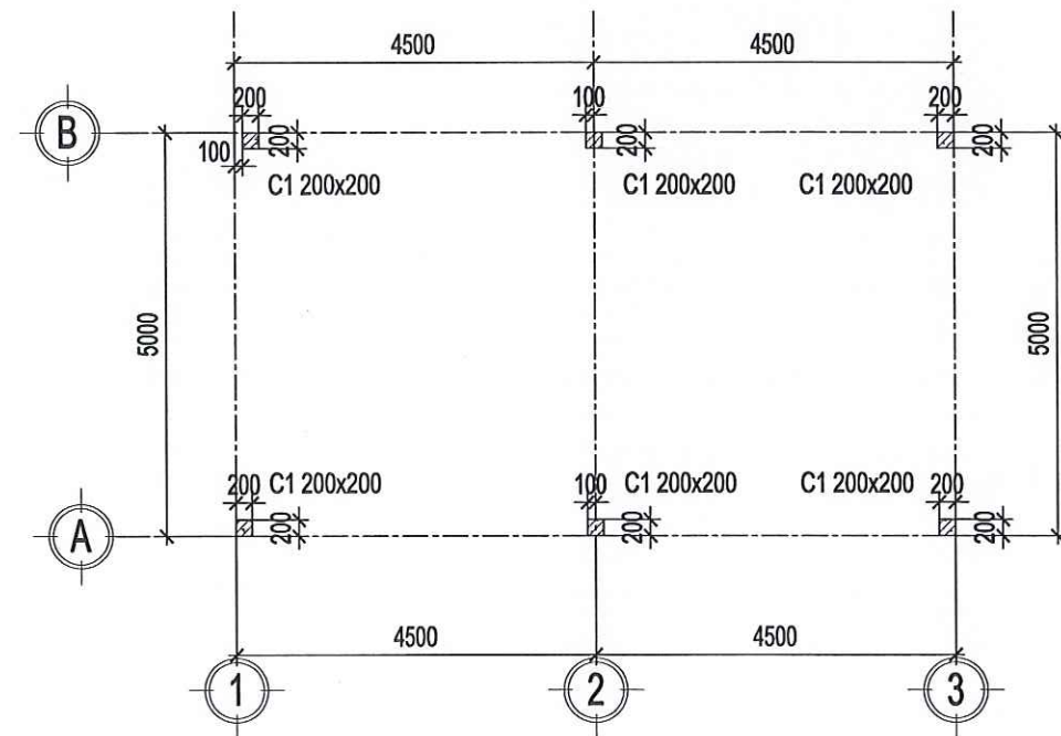
MẶT BẰNG CỘT TẦNG 2
