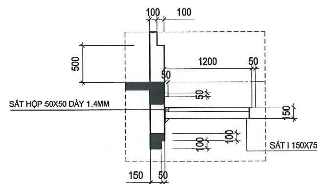
CHI TIẾT 7 TL:1/50
