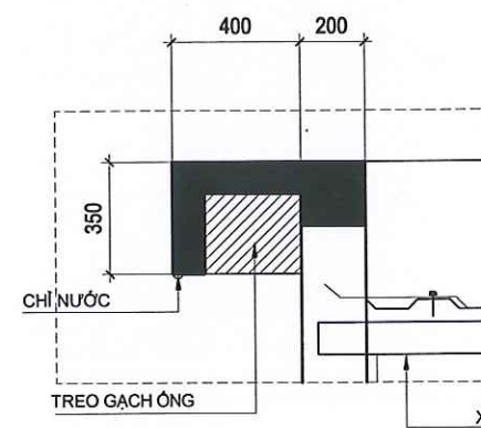
CHI TIẾT 15 TL:1/25
