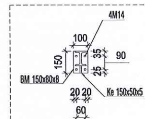
CHI TIẾT LIÊN KẾT MÁI CHE TL:1/25
